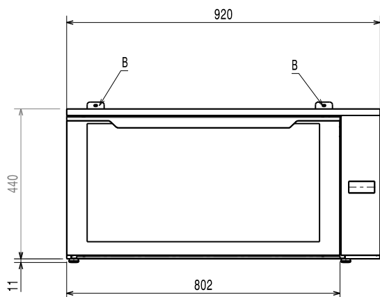
Zij aanzicht
